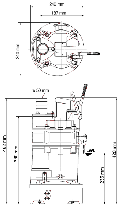
KTVE22.2-51
