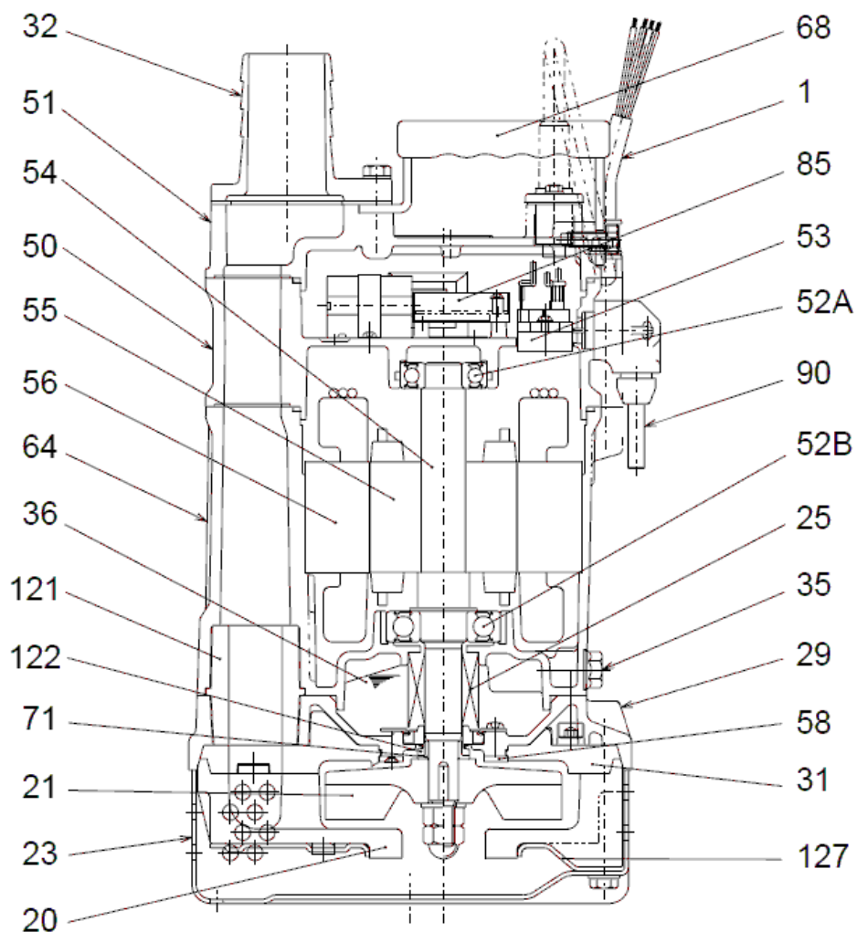
KTVE22.2-51
